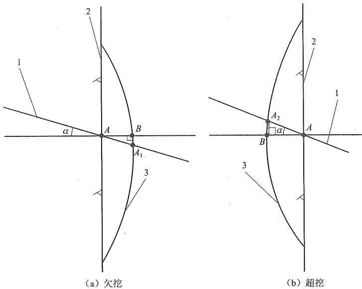
图 C.0.1 岩壁梁锚杆开孔位置与设计孔位关系图
